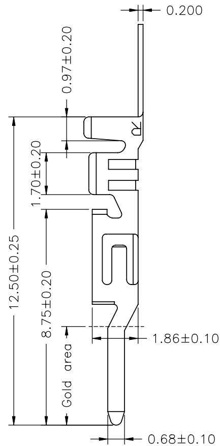
SEC:A-A
